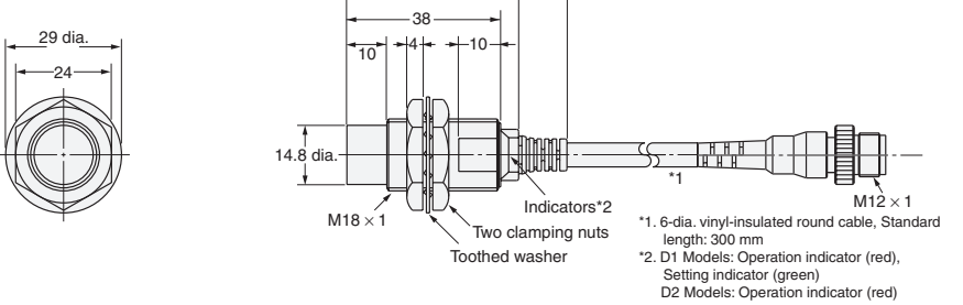
Diagram 32 E2E-X14MD□-M1GJ E2E-X14MD1-M1TGJ E2E-X14MD□-M1TGJ-US
