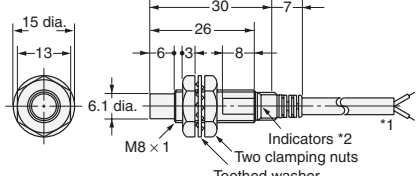
Diagram 2 E2E-X4MD□ E2E-X2ME□/F□
