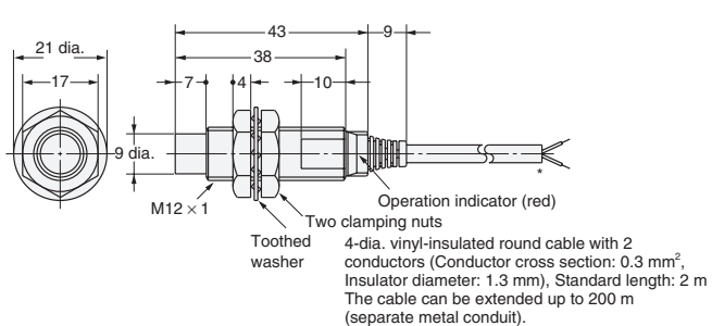
Diagram 8 E2E-X5MY□
